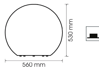
DORA L 2462-56 1x E27
