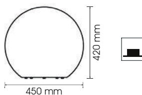
DORA M 2462-45 1x E27
