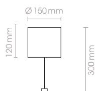
57314-15 230V · E27 · 40W
