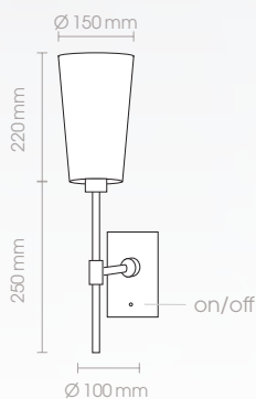
57230-16 230V · E14 · 40W
