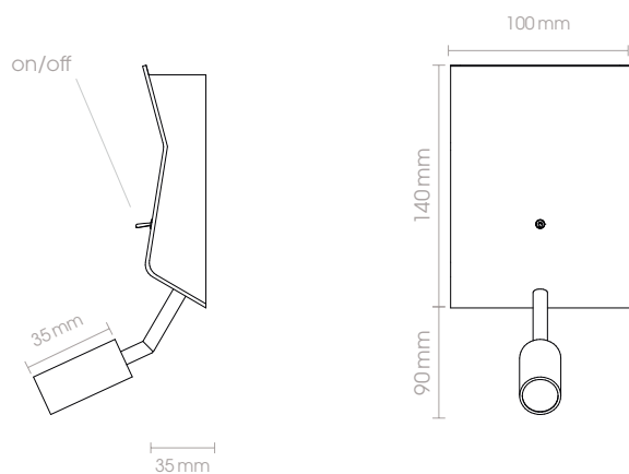
57204SP-03 57204SP-11 57204SP-16 30V · LED · 3W · 270lm · 3000K Leselicht LED · 2W · 180lm · 3000K
