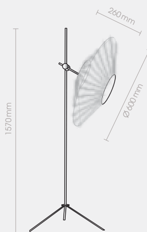
56663-45 230V · LED · E27 · 40W
