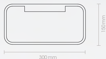
57203E-30 230V · LED · 5W 480lm · 3000K
