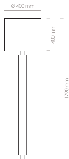
57310-40-PR 230V · E27 · 40W LED · 12W · 792lm
