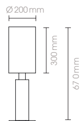
57309-20-PR 230V · E27 · 40W LED · 3W · 198lm
