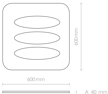
OC3561 230V · LED · 46W TW 4500 K · 2380lm WW 3000 K · 2160lm
