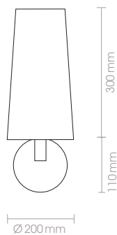
57222 230V · E27 · 40W
