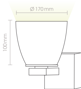
5303-09 230V · LED · 3W 280lm · 3000K A 137 mm
