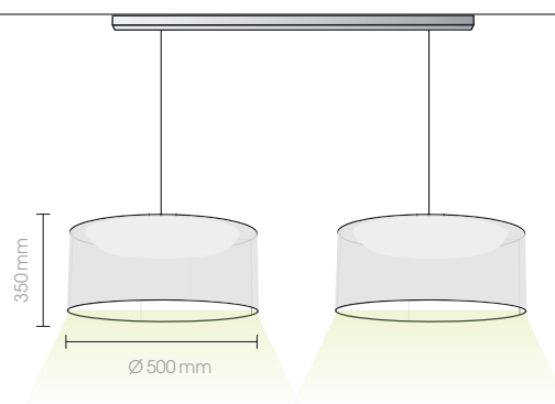
57017-2-50 230V · 2xE27 · 40W
