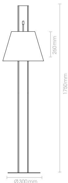
57321 230V · E27 · 40W LED · 17W · 1122lm · 3000K
