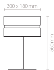
56332R-16 230V · E27 · 40W
