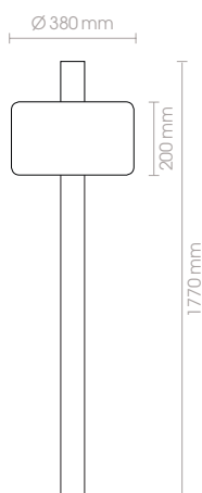
57324 230V · E27 · 40W LED · 17W · 1122lm · 3000K A 30mm
