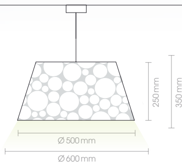
57028-50 230V · E27 · 40W
