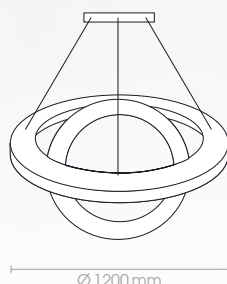
56574-2-120 230V · LED · 165W 12208lm · 3000K
