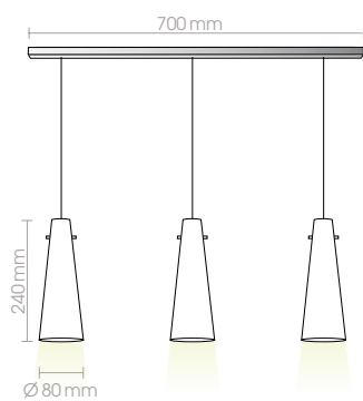
3958T-09/-11/-13/-16 230V · 3xE14 · 40W
