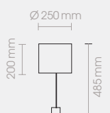
57305-25 230V · E27 · 40W
