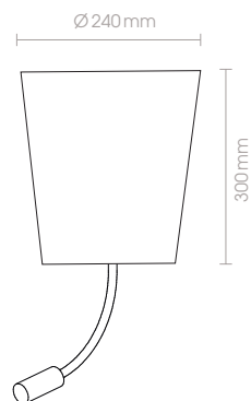
57207LA 230V · E27 · 40W Leselicht LED · 2W · 180lm
