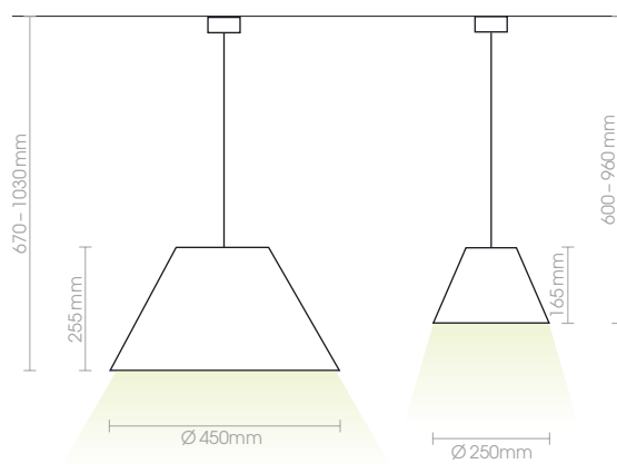
53123-19 230V · E14 · 40W
