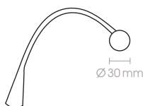
W5178-11 W5178-16 230V · LED · 2W · 180lm Lese-arm 410 mm
