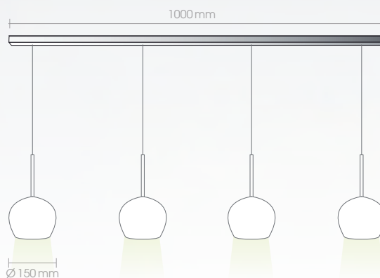
2278-4-15A/W 230V · 4xE14 · 40W
