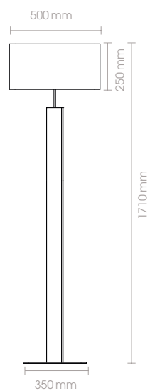
57326 230V · E27 · 40W LED · 14W · 792lm · 3000K A 20 mm
