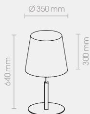
57337-35-03 57337-35-16 230V · E27 · 40W
