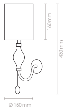
5295-09-PG3 230V · E14 · 40W
