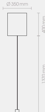
57312-35 230V · E27 · 40W
