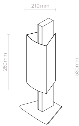
57306-21 230V · LED · 18W 2x675lm
