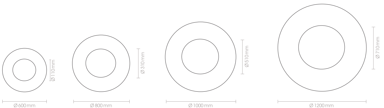
57225-60 230V · LED · 18W 1280lm · 3000K
