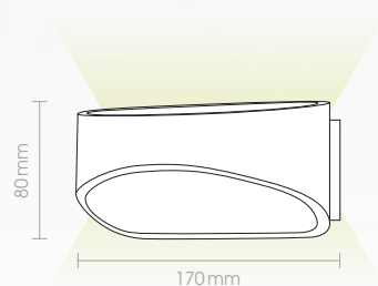
5304-09 230V · LED · 5W 480lm · 3000K A 100 mm
