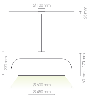
57061 230V · E27 · 40W
