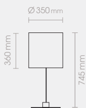
57304-35 230V · E27 · 40W
