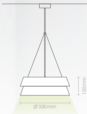
57030-33 230V · LED · 15W 1800lm · 3000K
