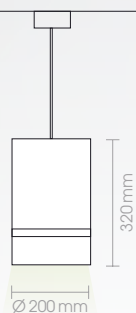
57022-20 230V · E27 · 40W
