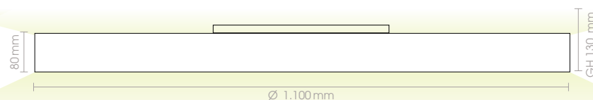
56717-110-80/V17 230V · 3xE27 · LED · 87W 16360lm · 3000K
