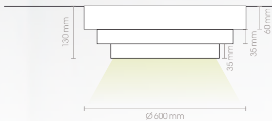
57135-13 230V · LED · 24W 4760lm · 3000K
