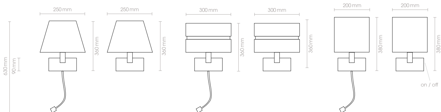
56331K-16-PG1 230V · E27 · 40W Leselicht LED · 2W · 180lm · 3000K
