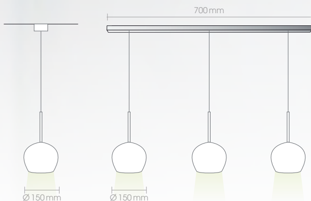
2278-09A/W 230V · E14 · 40W
