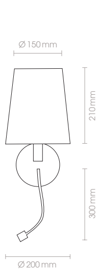
57234L 230V · E27 · 40W Leselicht LED · 2W · 180lm · 3000K
