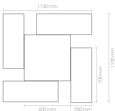
57115-110 230V · LED · 56W 9280lm · 3000K
