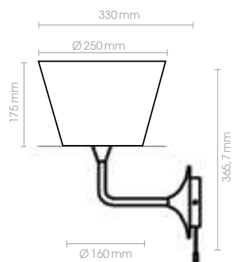
56346P-15 230V · E27 · 40W
