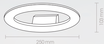
57203R-25 230V · LED · 7W · 580lm A 135 mm
