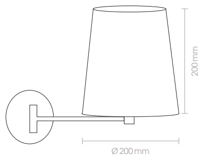
57236 230V · E27 · 40W
