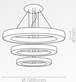
56574-3-90 230V · LED · 249W 18588lm · 3000K
