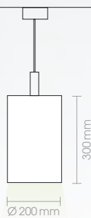
57068-20 230V · E27 · 40W
