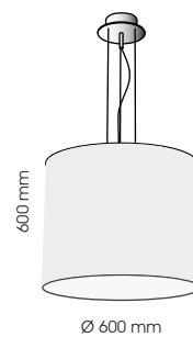
56393-60 230V 3x E27 LED
