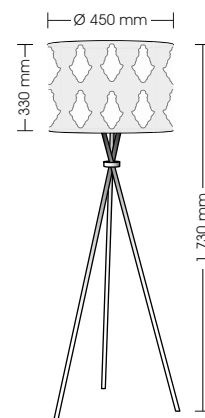
56672-45 230V 3x E27 LED
