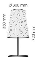
56683-30 230V 1x E27 LED
